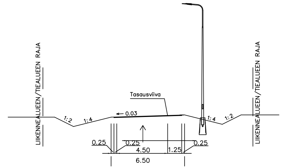
E1R1, E1R2, E1R3, E1R4A, E1R4B, E1R5, E3R3 ja E3R4 Peruspoikkileikkaus 6.5/4.5
